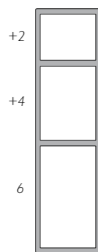
RGS 6+4+2
