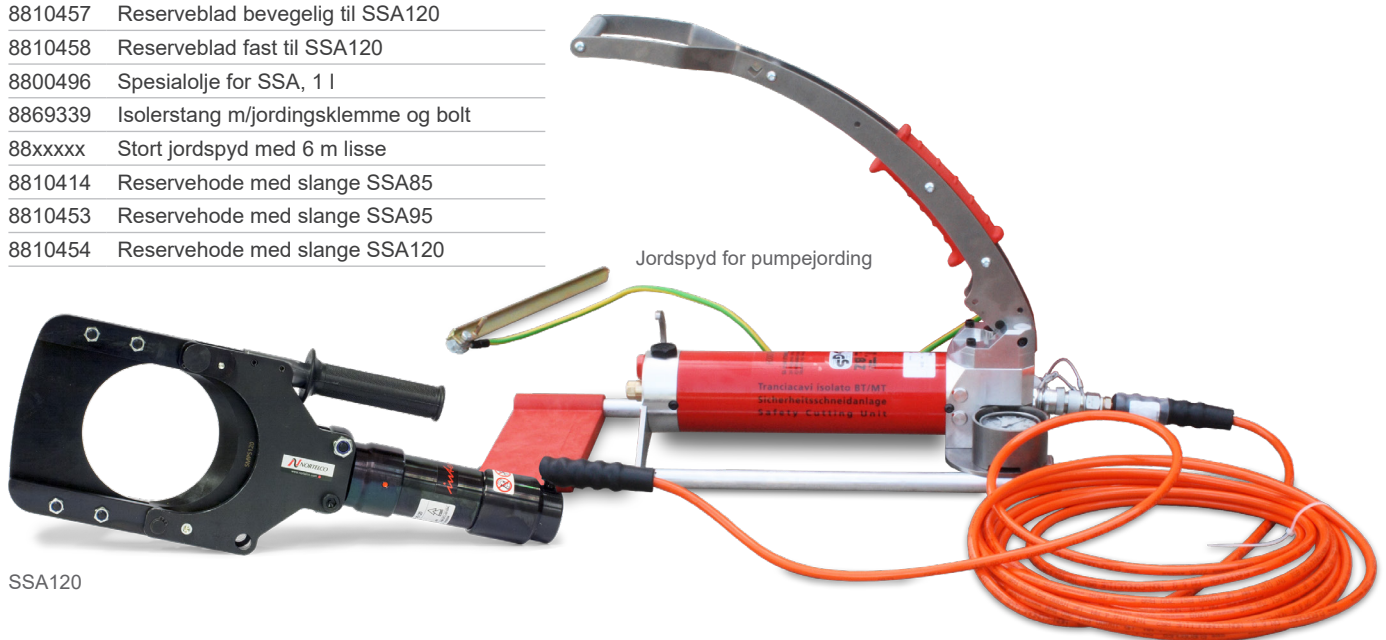
Stort jordspyd 1 m med lang lisse 6 m
