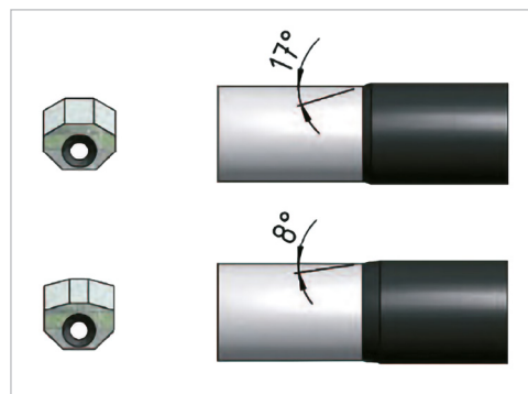
FBS 2 leveres med kniv for enten 17 eller 8 graders skjærevinkel.
