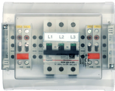
8210103 – MOK 230 S EPI
