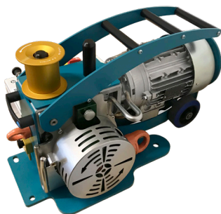
Elnr. 8854691 Elektrisk kabelvinsj for multibruk, med minihjul, 12 kN. Modell: JVM1200CAE
