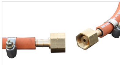
8810491/92 Tilkoblingsstusser/slangeklemmer
