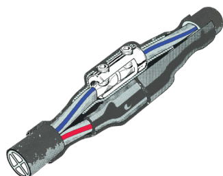
11 Lavspentskjøter
