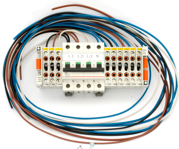
8210130 – MOK 400V TN-S EE m/kabel
