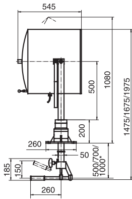
NHS550C Gewicht/ weight: 26.7 kg
