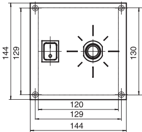
Steuergerät STG1/ control unit STG1 Gewicht/ weight: 0.3 kg
