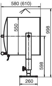
NHS550A Gewicht/ weight: 23.3 kg
