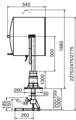
NHS550D Gewicht/ weight: 32.0 kg
