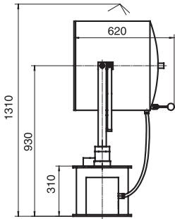
NHS550F Gewicht/ weight: 48.0 kg
