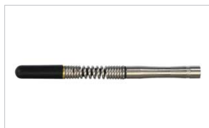
Elnr. 8854660-63 Lokaliserbare sonder for trekkefjærer, finn blokkeringer og skader i rør \varnothing 6-16 mm. Modell: VMSS336 ++
